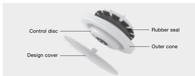
ComfoValve Luna E, Explosionszeichnung
